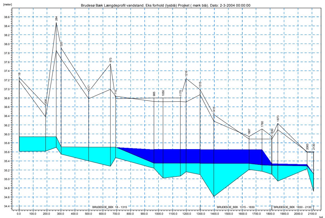
Figur 4 Brudesø Bæk Længdeprofil vandstand. Vandstand vinter ved moderat afstrømning. Lys blå eks. forhold og mørk blå viser vandstandshævning efter anlæg af overløbsbygværk ved Holm vej.
