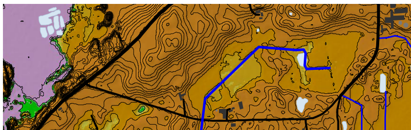
Figur 11 Brude Sø st. 1740. Vandføring eks. forhold (sort) og efter anlæg af overløbsbygværk ved Holmvej (blå).
