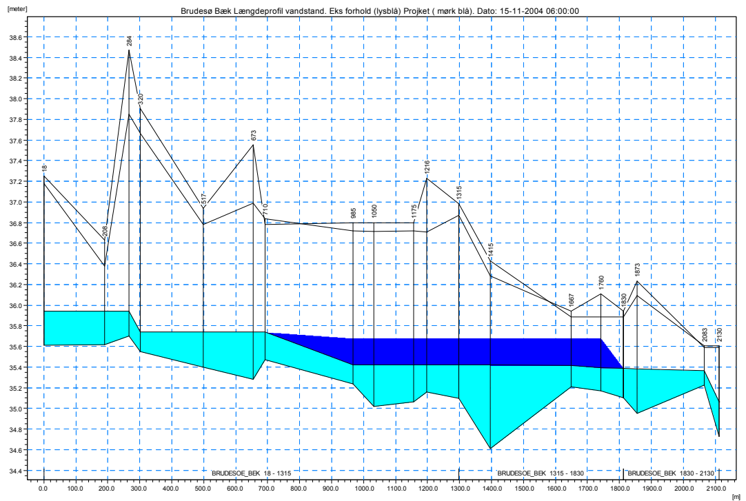
Figur 7 Brudesø Bæk Længdeprofil vandstand. Vandstand efterår høj afstrømning ( Brudesø under opfyldning). Lys blå eks. forhold og mørk blå viser vandstandshævning efter anlæg af overløbsbygværk ved Holm vej.
