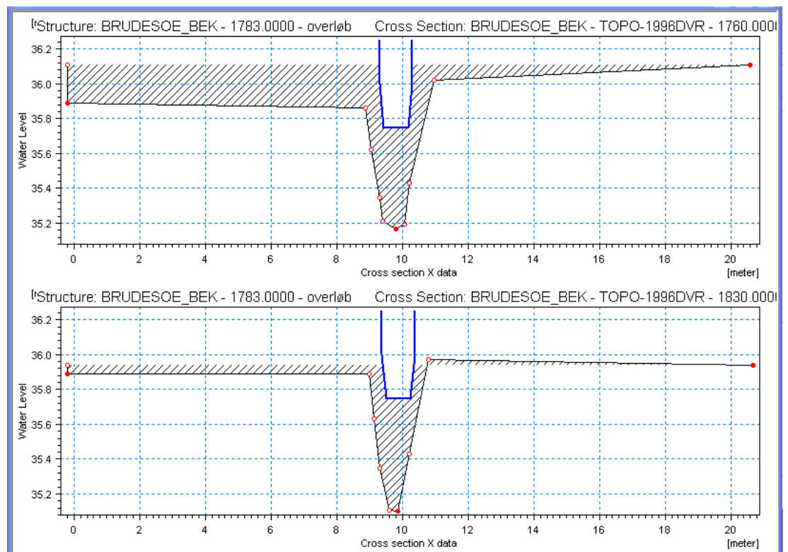
Figur 2 Overløbsbygværk i Brudesø Bæk ved Holmvej. Overløbskote: 35.75 DVR90
