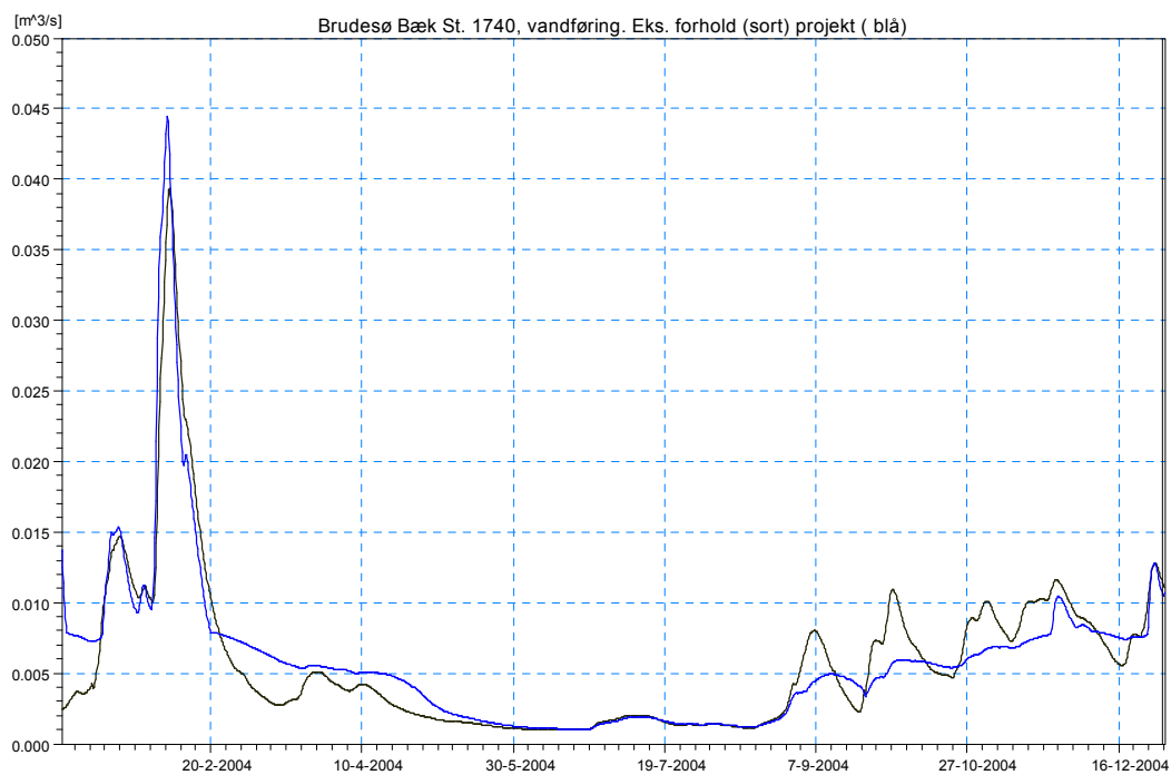
Figur 11 Brude Sø st. 1740. Vandføring eks. forhold (sort) og efter anlæg af overløbsbygværk ved Holmvej (blå).
