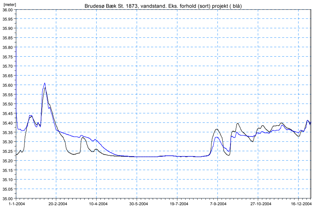
Figur 10 Brude Sø st. 1873. Vandstand eks. forhold (sort) og efter anlæg af overløbsbygværk ved Holmvej (blå).
