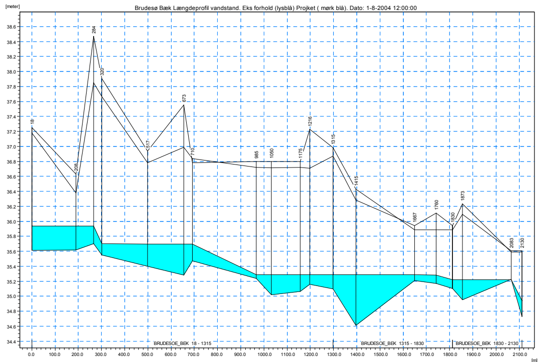
Figur 6 Brudesø Bæk Længdeprofil vandstand. Vandstand sommer ingen afstrømning. Vandløbet er tørlagt på store dele af strækningen (Dette kan dog ikke vises i M11 modellen idet modellen kun kan foretage beregninger med vand i vandløbet).
