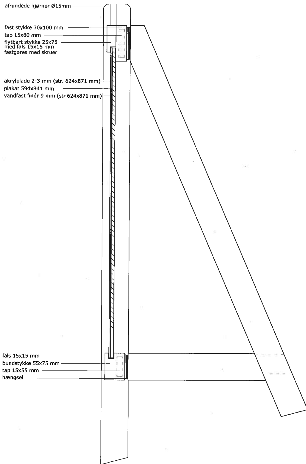
lodret snit i skilteflade
