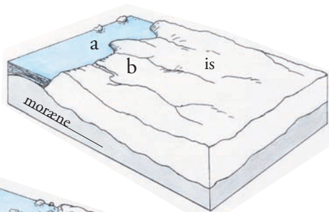
Tre stadier af landskabets udformning ved Vissenbjerg bakke og konsolbakken ved Bred. Omtegnet efter Aksel Schou (1949) og Johannes Krüger (2000).
