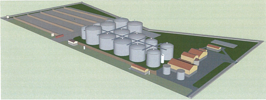
Figur c. 3D model af biogasanlæg
