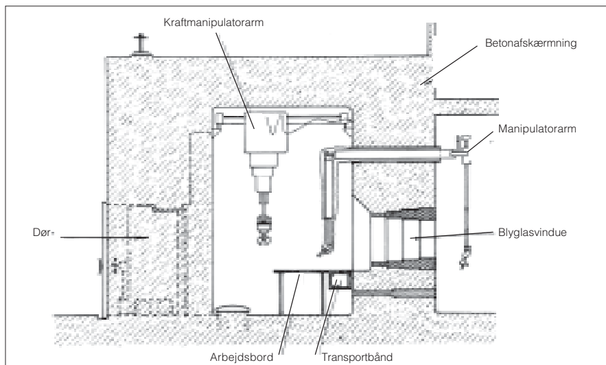
Figur 4.17 Lodret snit gennem en betoncelle med manipulatorarme og betonskærmning.
