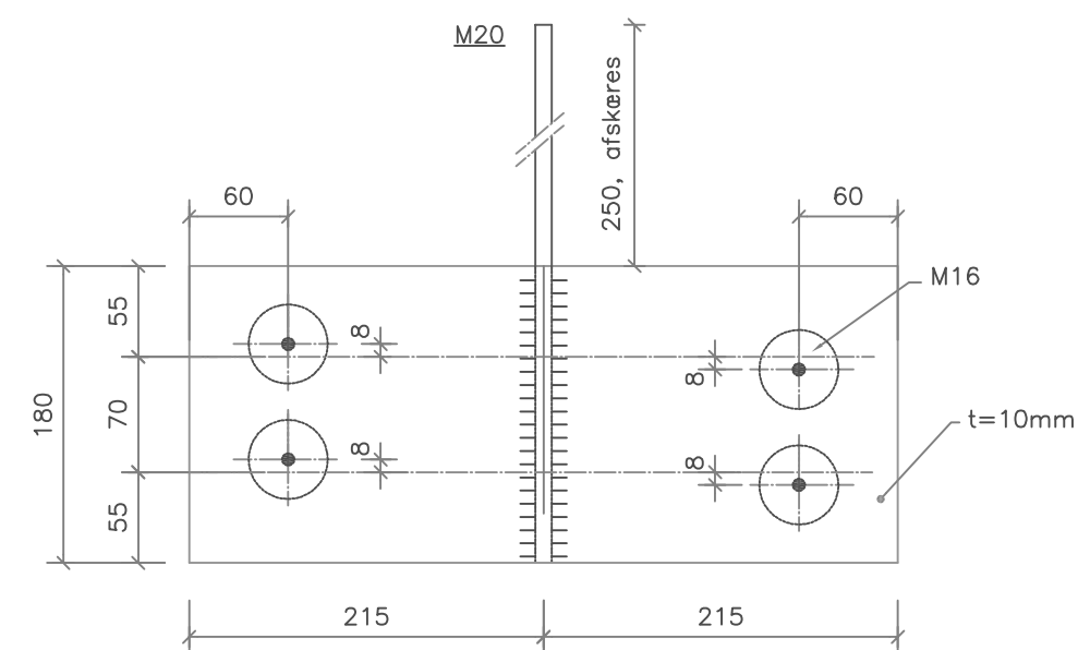
Type 6, bræddetag Type 6-2, bræddetag
